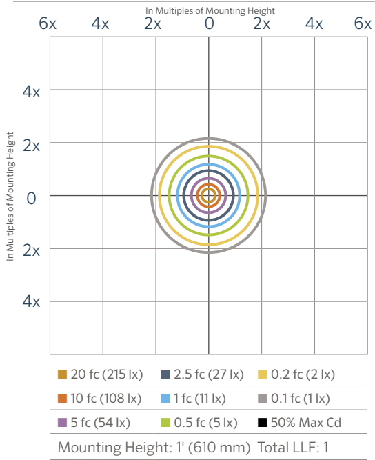
TD ZDC Isofootcandle Plot
